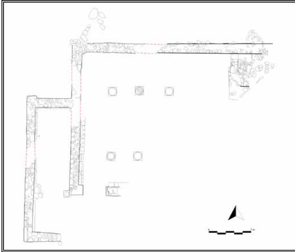
Figür 11: Bazilikal Planlı Kilisenin Birinci Evreye Ait Planı
