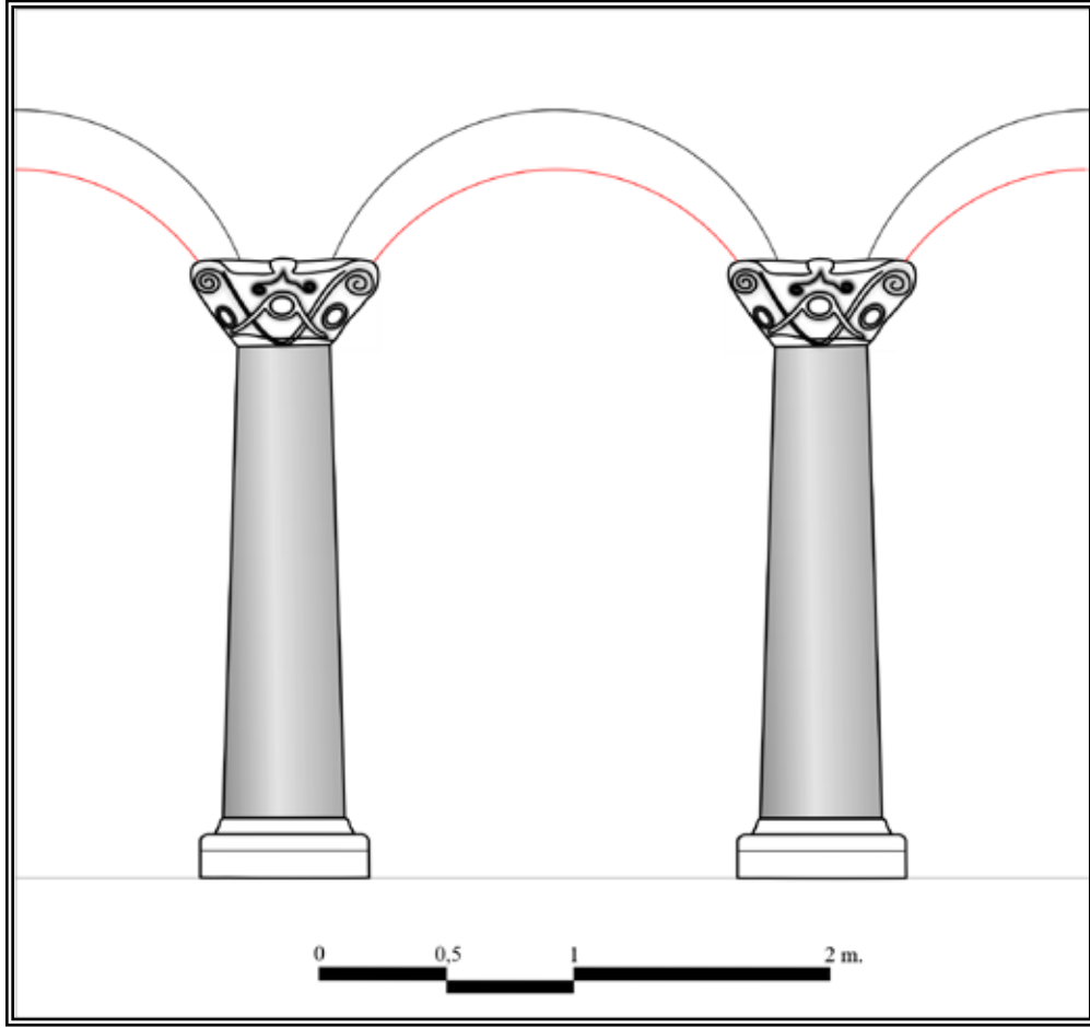
Figür 13: Bazilikal Planlı Kilisenin Birinci Evresine Ait Destek ve Bağlayıcı Sisteminin Restitüsyonu
