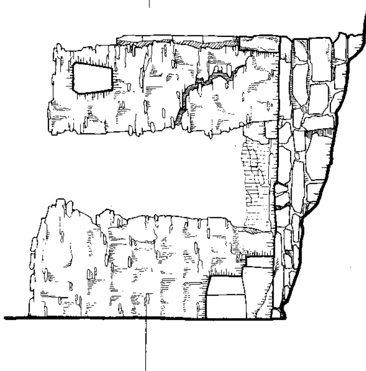
დარბაზის ფასადი მ-1:25
